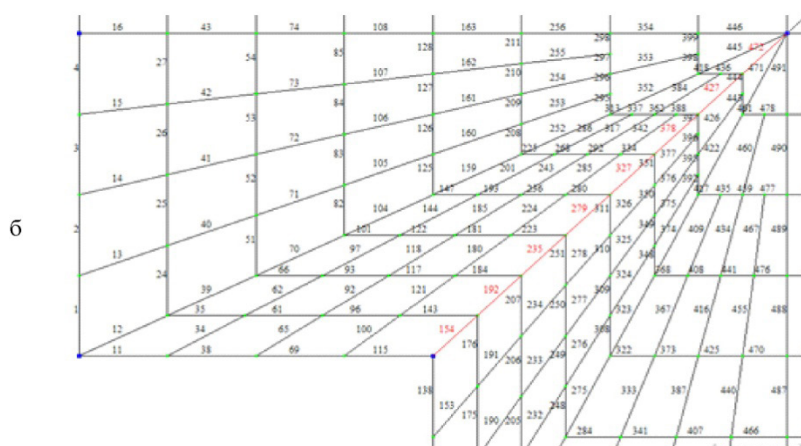
Рисунок 6 – К расчету радиального ребра: а – фрагмент расчета сечения ребра; б – красным цветом выделен элемент № 154
