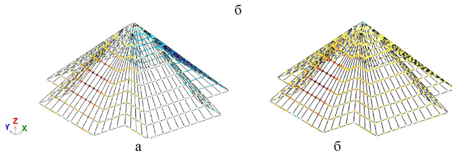
Рисунок 4 – Мозаика перемещений по оси X
