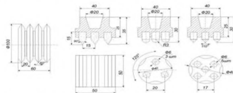
Рис. 3. Инструмент для фактурной обработки природного камня.
