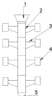
Рис. 2. Блок отливок: 1- литниковая чаша; 2- стояк; 3- питатели; 4- отливки; 5- зуппф.
