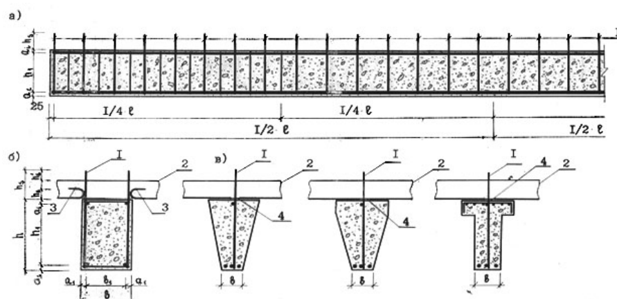
Рисунок 2 – Конструкция сборного железобетонного прогона:
