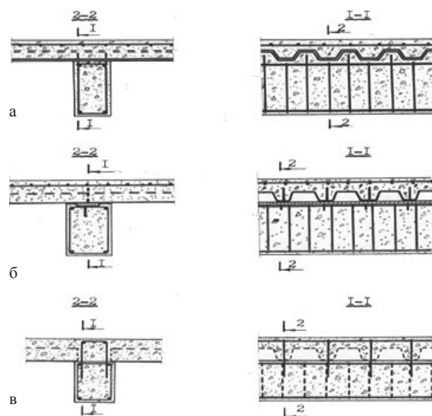
Рисунок 1 – Конструкции перекрытий, возводимых по железобетонным прогонам: а – по часторебристым прогонам; б – по прогону с металлической полоской по верхней грани; в – по прогону с петлевыми хомутами-анкерами
