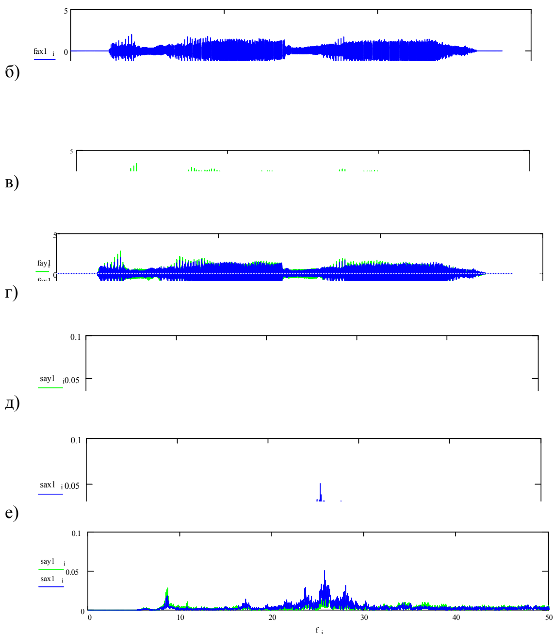
Рис. 7. Запись сейсмического воздействия на модель подпорной стенки, экспериментальные данные:
