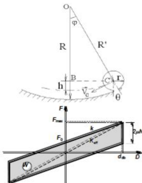
Рис. 2. Расчетная схема инерционного демпфера
